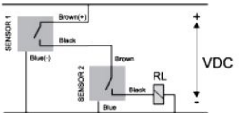
سه سیمه PNP
