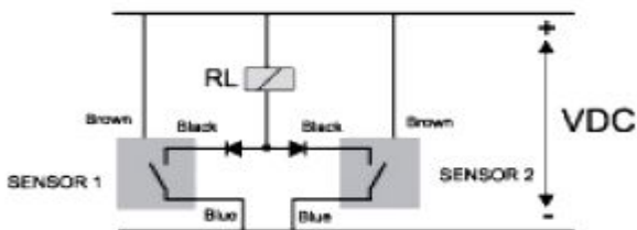
سه سیمه NPN
