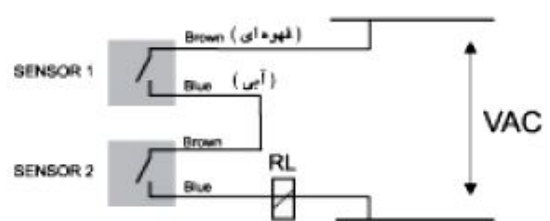
دو سیمه AC ( تعداد سنسور مجاز حداکثر دو عدد می تواند باشد. )
