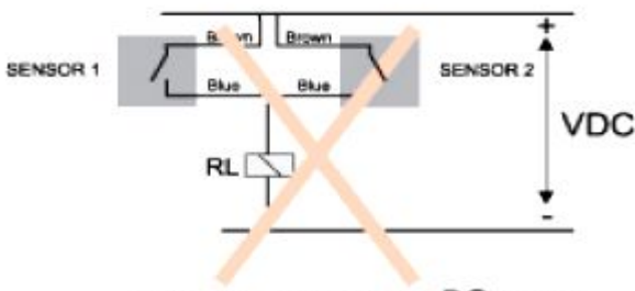
دو سیمه DC ( اتصال موازی مجاز نمی باشد. )
