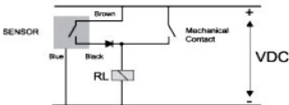
سه سیمه PNP موازی با کنتاکت مکانیکی
