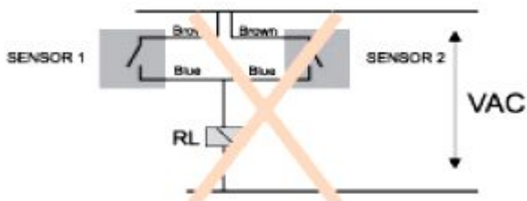
دو سیمه AC ( اتصال موازی مجاز نمی باشد. )
