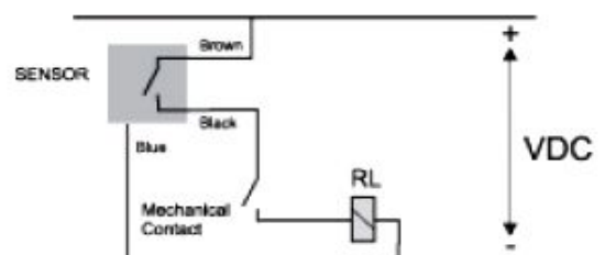
سه سیمه PNP سری با کنتاکت مکانیکی
