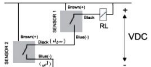
سه سیمه NPN
