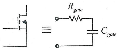
مدل ساده شده برای محاسبه تلفات گیت. n-1۰ ک ۴
