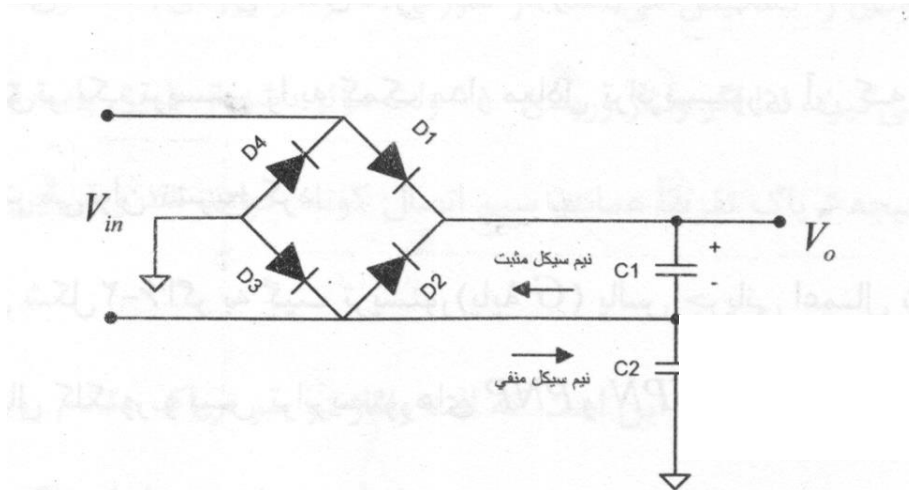
شکل B-3- وضعیت مدار دلتا به ازای ولتاژ ورودی ۱۱۰ ولت مؤثر
