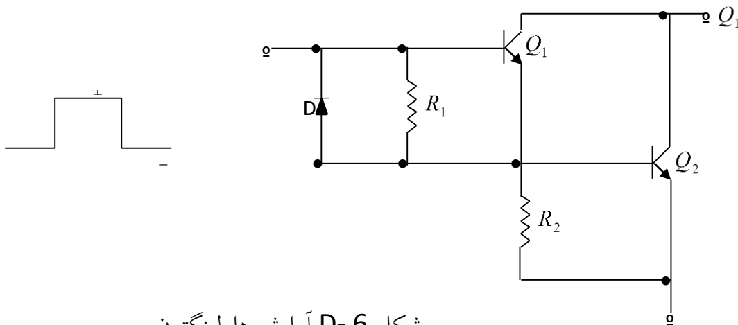
شکل 6- D آرایش دارلینگتون
