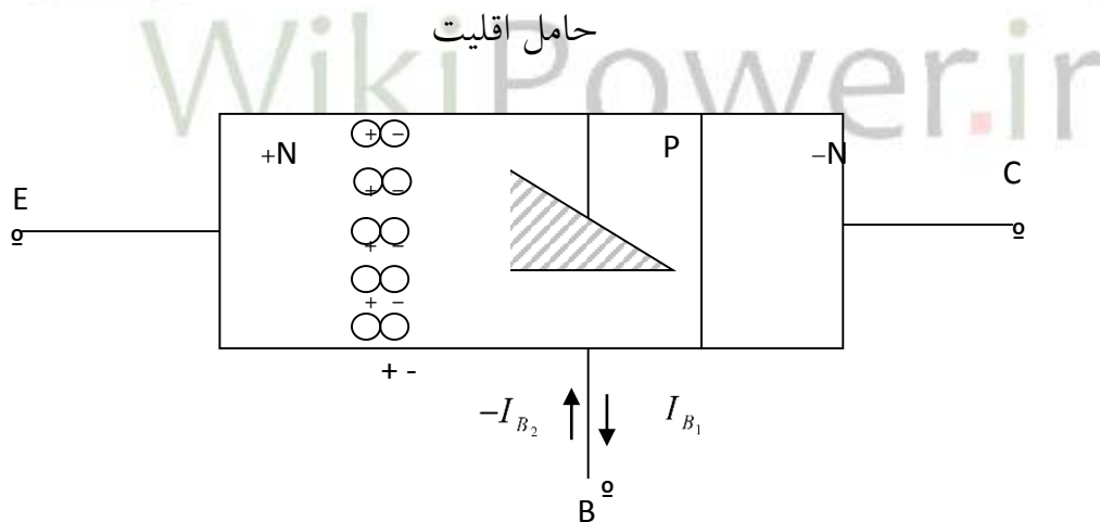
شکل D-1 شمای داخلی یک ترانزیستور دو قطبی NPN
