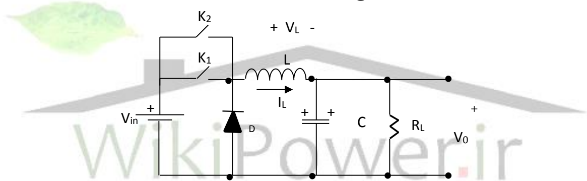
ساختار مبدل پوش - پوش غیر ایزوله
