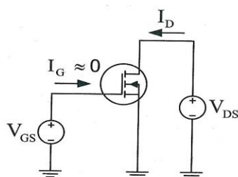
شکل D-10: جریان در ترانزیستور ماس فت در حالت استاتیکی.
