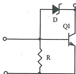
شکل D-9 مدار شاتکی TTL جهت افزایش سرعت در مدارهای TTL
