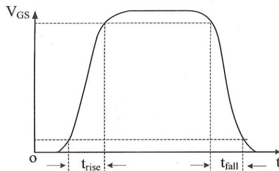
شکل D-12 تغییرات ولتاژ گیت ترانزیستور ماس فت.
