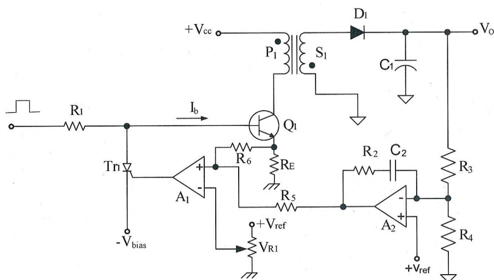
نمایش مبدل مد ترکیبی.
