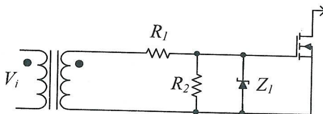
شکل D-8 نمونه ای از مدار راه انداز گیت ترانزیستور ماس فت. ۱ . Gating Loss
