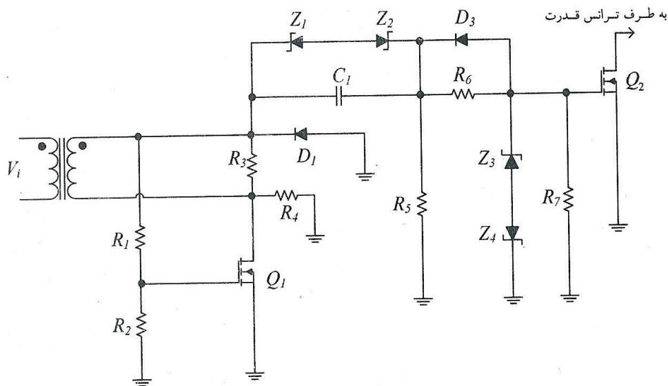
نمونه‌ای دیگر از مدار راه‌انداز گیت مناسب برای قدرت و فرکانس زیاد. n-۵ ک ۴
