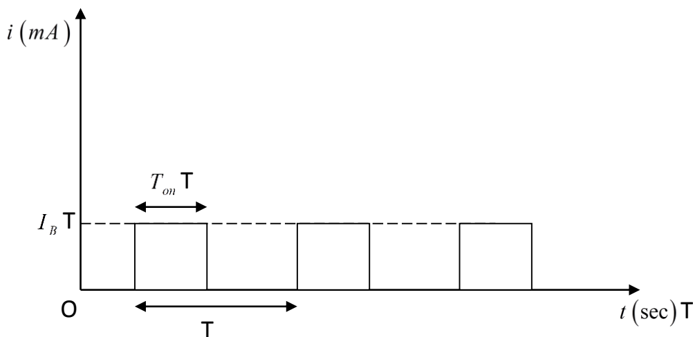
شکل D-1 پالس غیرمناسب جهت راه اندازی بیس ترانزیستورهای دو قطبی
