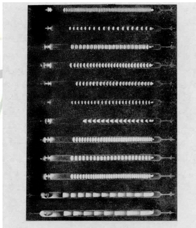
شکل (۱۰)-حالت های مختلف تخلیه روشن
