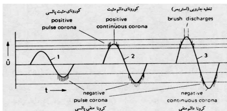
شکل (۱۶) - تخلیه جزئی یا کرونا در ولتاژ متناوب
