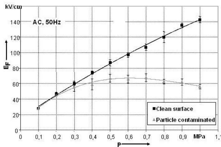
شکل ۴- استقامت میدان تخلیه سطحی مخلوط گازهای N_2 ۹۵٪ SF_6 ۵٪ فشار مطلق
