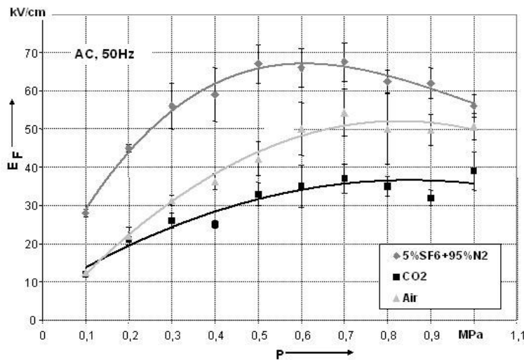
شکل ۵- استقامت میدان تخلیه سطحی مخلوط گازهای N_2 ۹۵٪ SF_6 ۵٪ فشار مطلق
