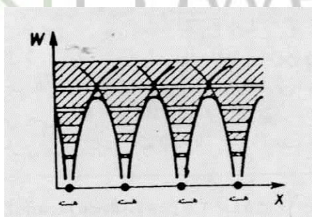
شکل (۷)- اتم های کریستال و سطوح انرژی آنها
