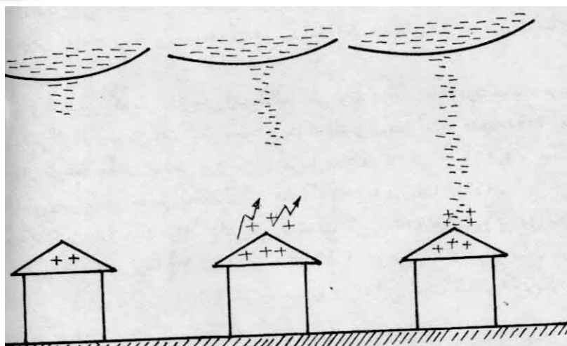
شکل (۲۷) - پیشرفت کانال هادی به طرف زمین و یونیزه شدن هوا در نقاط نوک تیز و مرتفع
