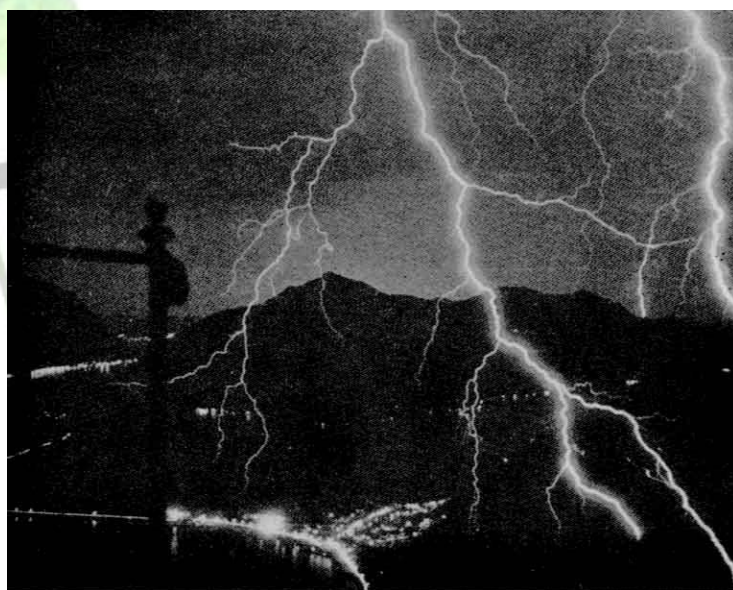
شکل (۲۸) - صاعقه با دو کانال اصلی
