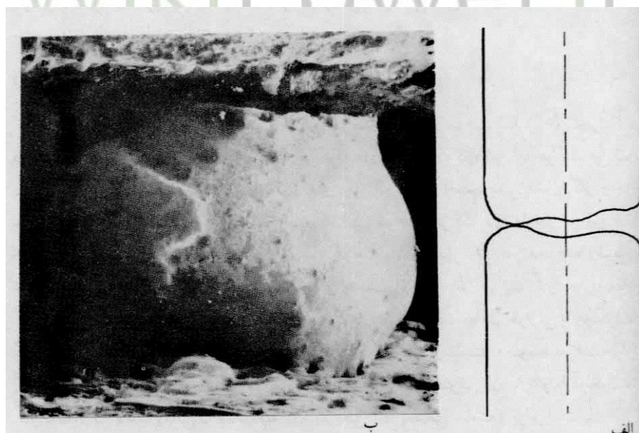
شکل (۲) - (الف) دو کنتاکت کلید در لحظه جدا شدن و (ب) ذوب شدن کنتاکت ها
