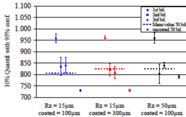
شکل ۱۲-۱۰. مقادیر با کمربند اطمینان از شکست اول و ولتاژ L1- منفی ضخامت پوشش متغیر و R_{z,s}=40\text{mm}
