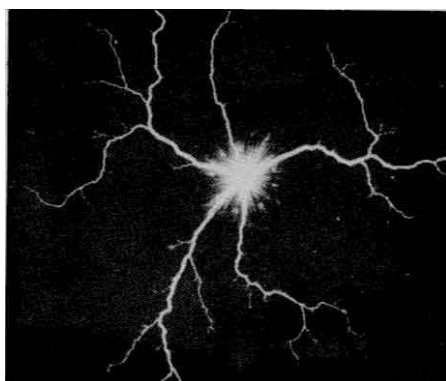
شکل (۲۵)- شکلهای لیشتنبرگ در هوا (ولتاژ ضربه مثبت)
