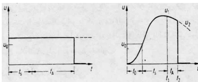
شکل (۲۹) - (الف) زمان تاخیر شکست در ولتاژ پله ای و (ب) در ولتاژ ضربه
