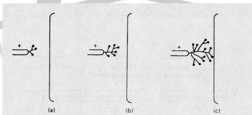
شکل (۱۷)-پیشرفت استریم در نوک سوزن در ولتاژ ضربه در طول زمان
