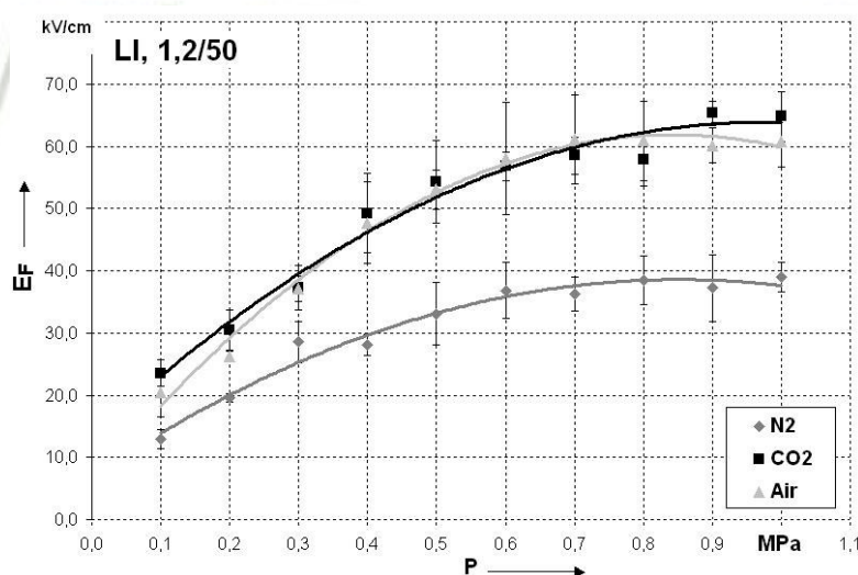
شکل ۳- استقامت میدان تخلیه سطحی فشار برای هوای فشرده و N_2 و CO_2 (با آلودگی ذره ای)
