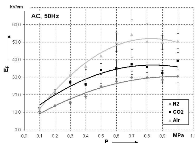
شکل ۲- استقامت میدان تخلیه سطحی فشاربرای هوای فشرده N 2 و CO 2 (با آلودگی ذره ای)
