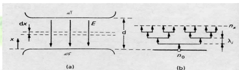
شکل (۶) - مدل تصویری افزایش الکترون ها و یون ها بر اثر برخورد
