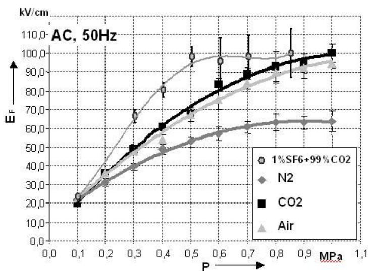
شکل ۱- استقامت میدان تخلیه سطحی فشاربرای هوای فشرده N 2 و CO 2
