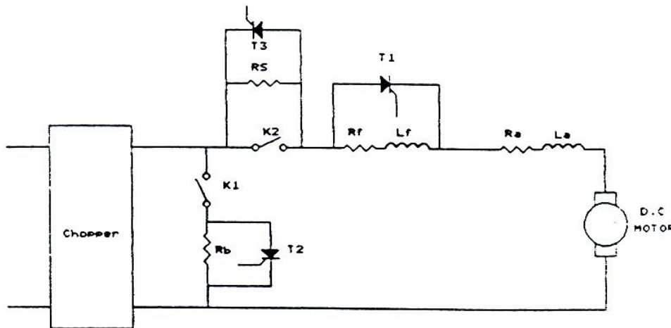
شکل (۳-۷) یک نمونه مدار کنترل چاپر ترکیبی
