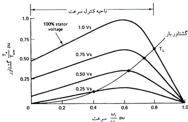
شکل (۴-۵) منحنی گشتاور- سرعت برای ولتاژهای متفاوت استاتور
