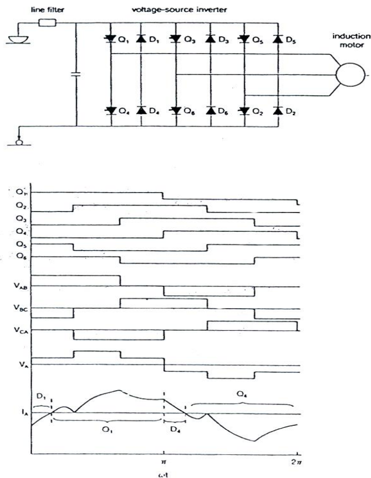
شکل (۵-۶) اینورتر منبع ولتاژ مدار قدرت و شکل موج ها
