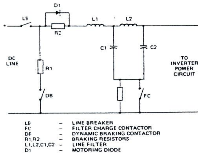
شکل (۵-۲) فیلتر ورودی، کنتاکتورها و مقاومت ها
