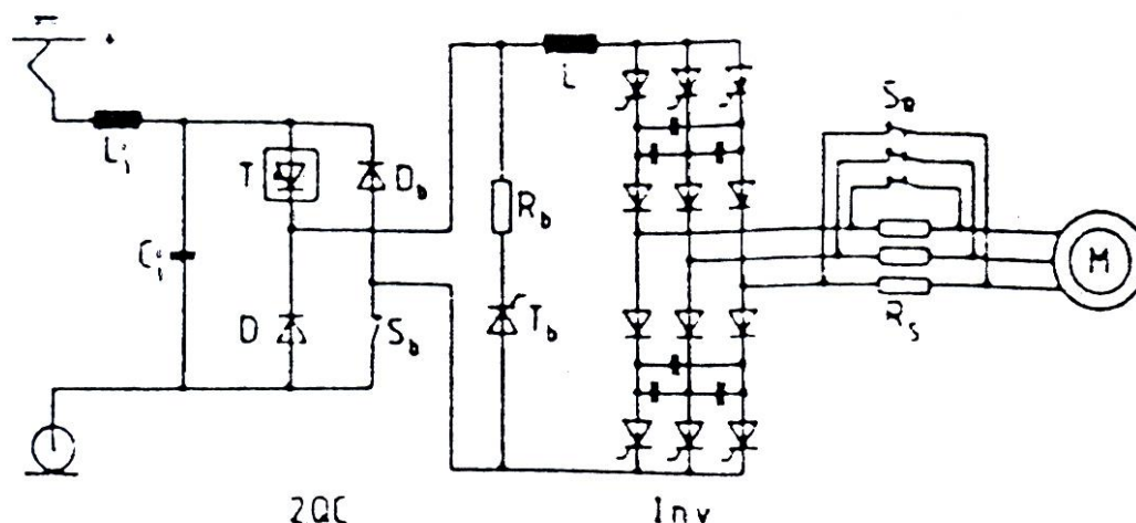
شکل (۶-۳) سیستم اینورتر منبع جریان با تغذیه DC
