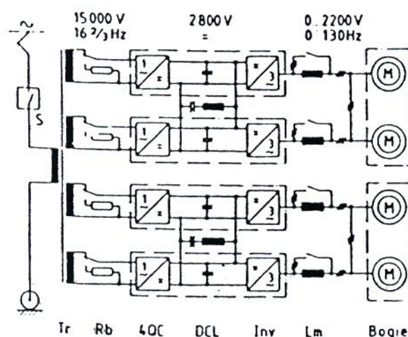
شکل (۶-۸) سیستم نیرو محرکه لوکوموتیو BR120
