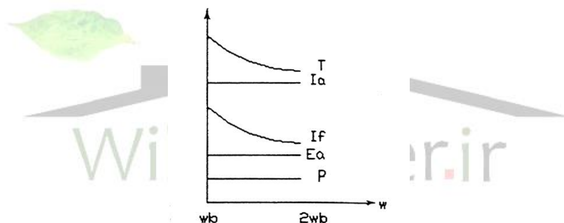
شکل (۵-۲) منحنی مشخصه های ژنراتور در حالت توان ثابت در ناحیه اول
