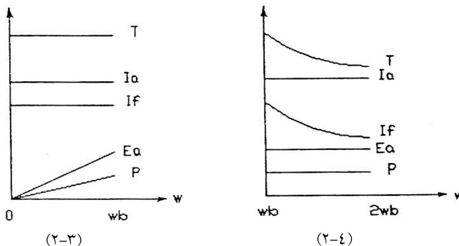
شکل (۲-۳) منحنی مشخصه های موتور در ناحیه اول
