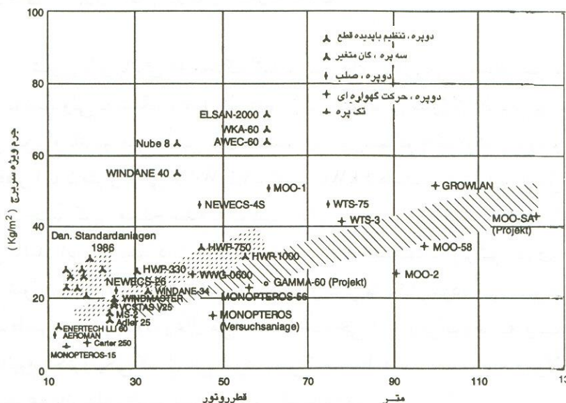
شکل ۳-۶ نمودار جرم مخصوص سر برج در مقابل قطر روتور برای توربینهای
