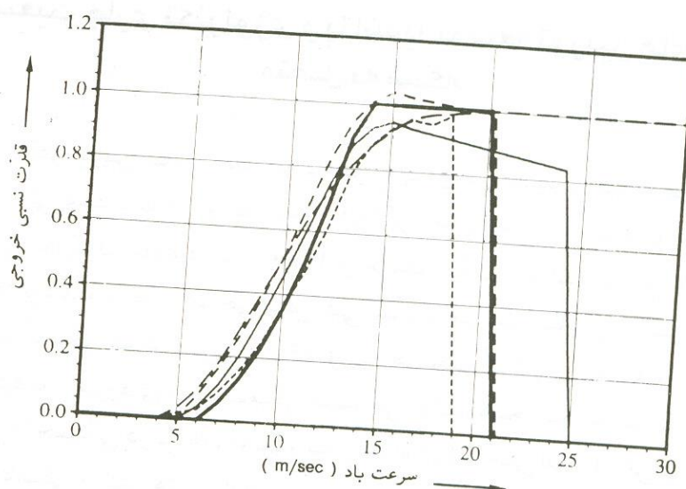
شکل ۵-۳ نمودار توان خروجی نسبی در مقابل سرعت باد برای توربین های جدید
