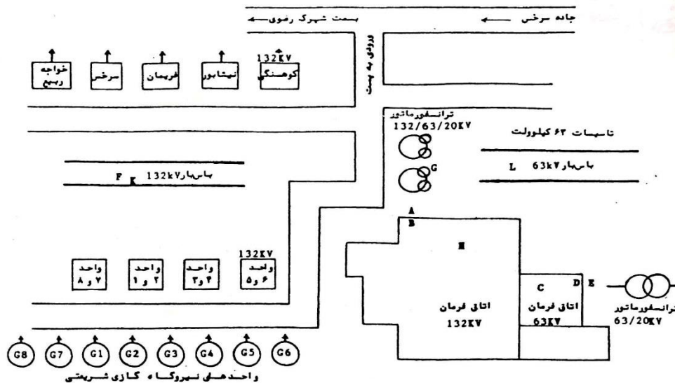
شکل ۲- فیروگاه و پست ۱۳۲/۶۳/۲۰ kV شریعتی
