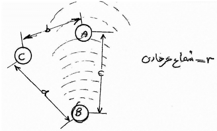
شکل (2-2) ضریب القاء خط سه فاز
