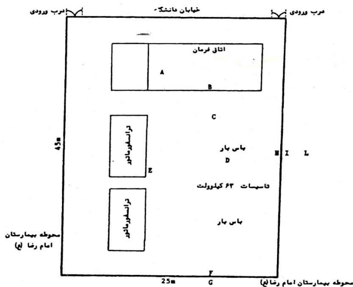
شکل ۳ پست ۱۳۲/۶۳/۲۰ kV امام رضا (ع)
