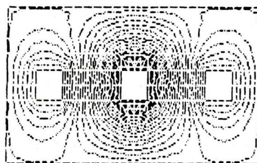
شکل ۳: خطوط هم پتانسیل مغناطیسی در لحظه Wt=210^\circ
