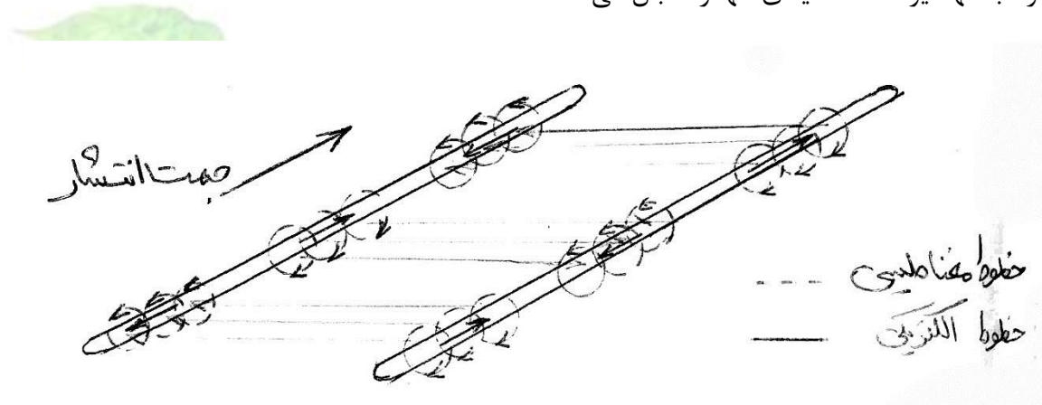
شکل ۳: امواج متحرک روی یک خط انتقال باز
