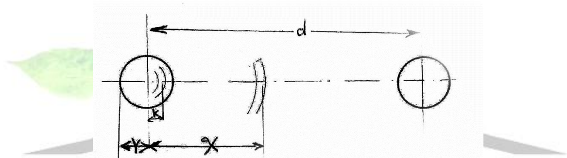
شکل ۱- ضریب القاء خط هوایی
