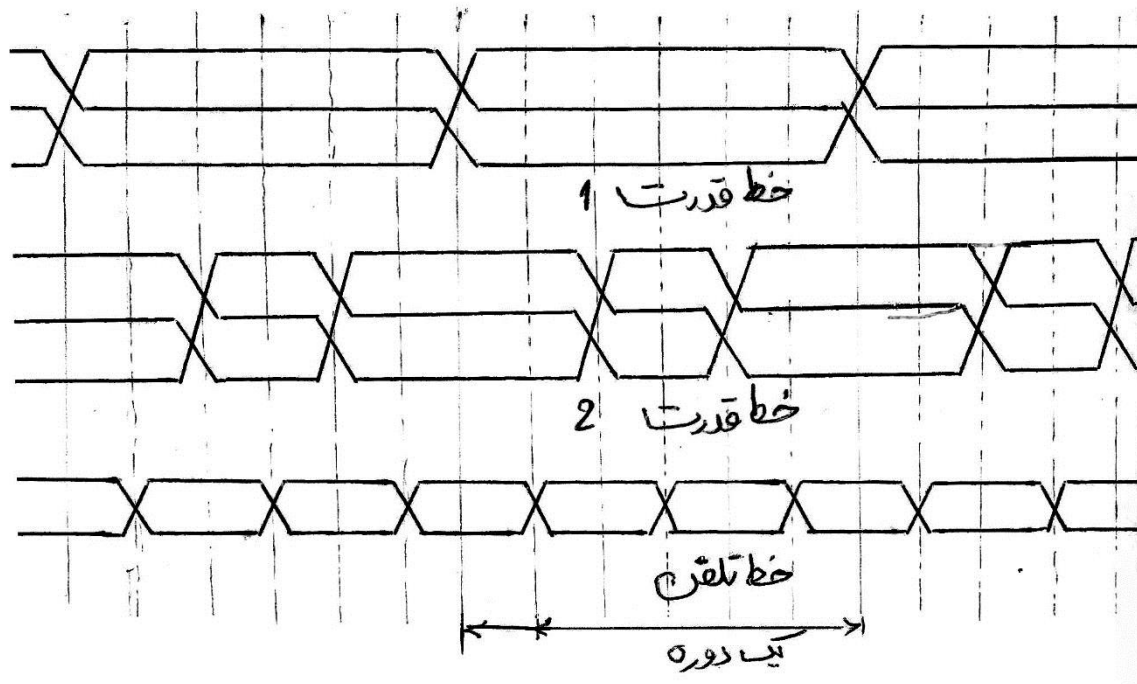
شکل ۴-۴- نمودار جابجا کردن دو خط قدرت و یک خط تلفن
