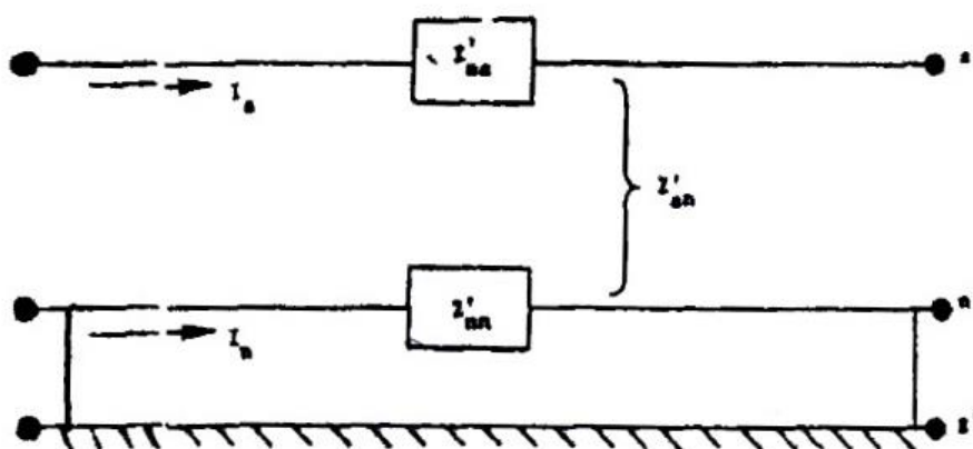
شکل (4-6) قسمت خط تکفاز
