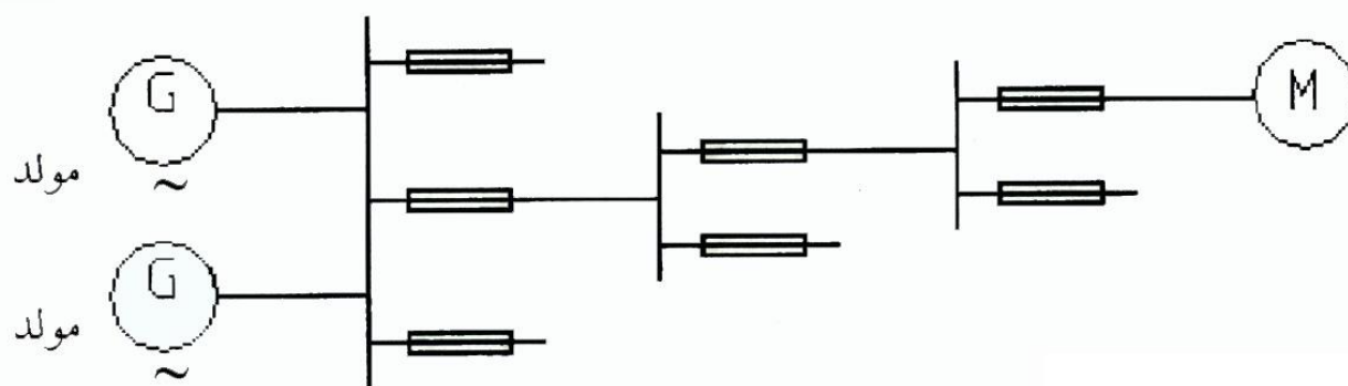
شکل (1-3) شبکه باز یا شعاعی (رادیال)
