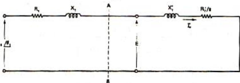
(ج) مدار معادل فاز ساده شده رجوع شده به استاتور
