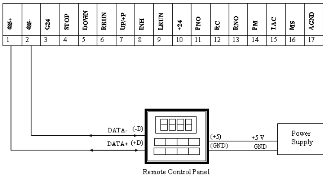
شکل ۸-۶: طرز اتصال پانل کنترل از راه دور به دستگاه
