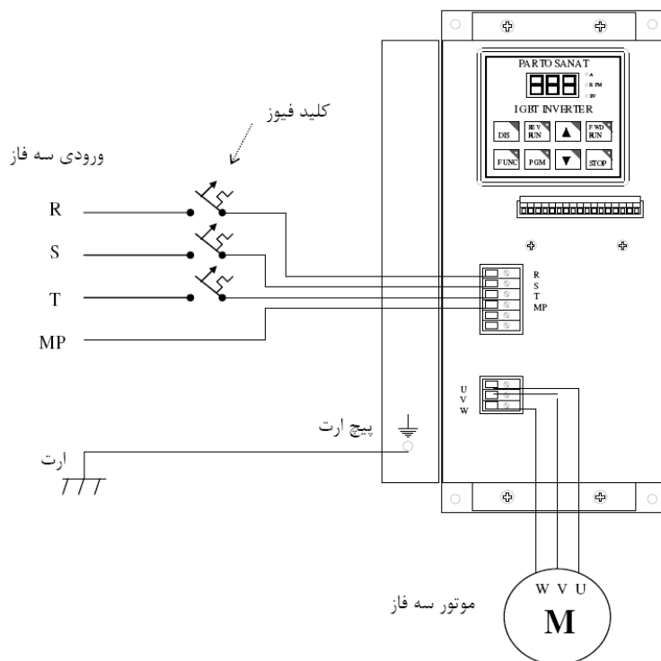
شکل ۲-۲: طریقه اتصال کابل های ورودی و خروجی به دستگاه
