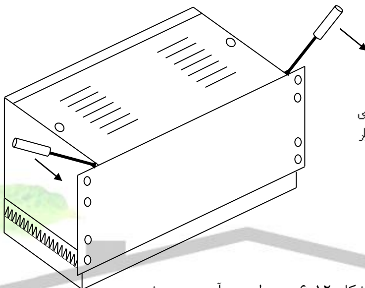
شکل ۱۲-۶: طرز در آوردن درپوش
