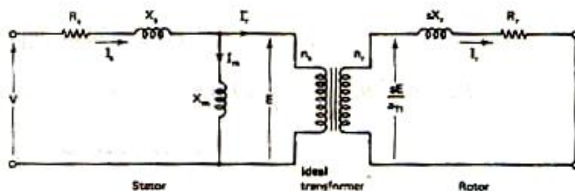
(الف) مدار معادل در فاز
