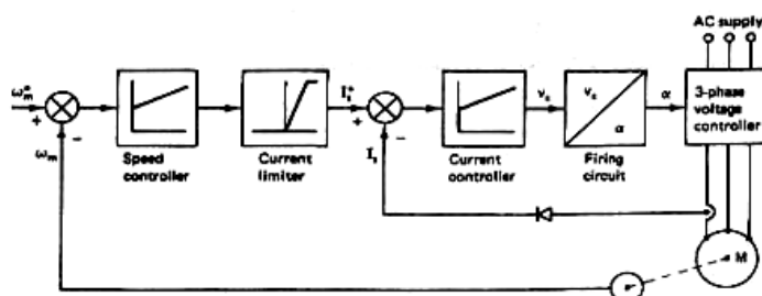
شکل ۵-۶ کنترل سرعت حلقه بسته تک ربعی
