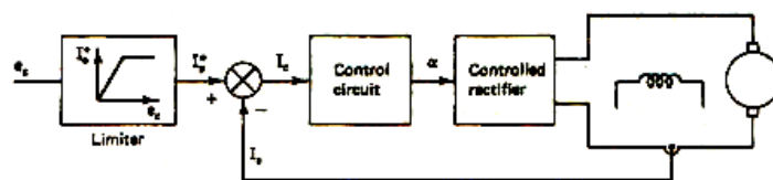
(الف) کنترل با حلقه داخلی جریان
