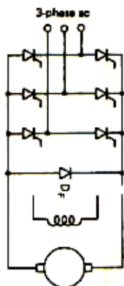
(ا) یکسوکننده ۶ پالسه
