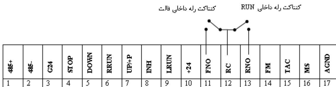
شکل ۶-۶: رله RUN و رله فالت داخلی دستگاه
