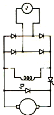
(ب) یکسوکننده ۲ پالسه
