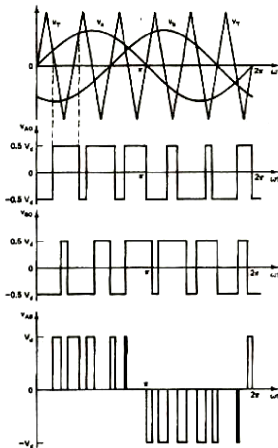
شکل ۵-۷ مدولاسیون پهنای پالس سینوسی
