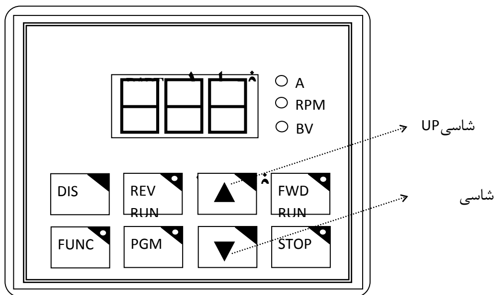
شکل ۳-۲: پانل کنترل دستگاه PSMC-DM
