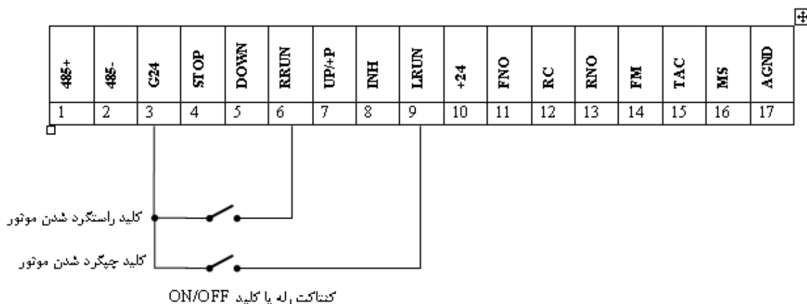
شکل ۴-۶: طرز اتصال کلید ON/OFF یا کنتاکت رله به ترمینالهای کنترلی
