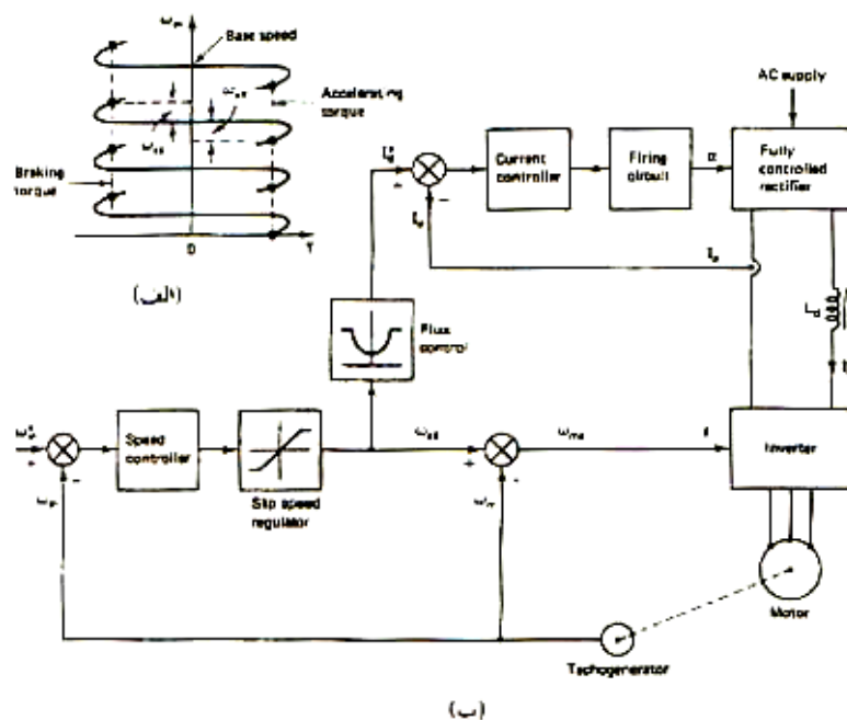
شکل ۷-۹ محرکه فرکانس متغیر CSI با کنترل سرعت لغزش
