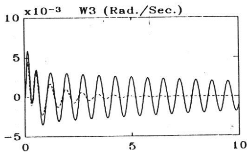
شکل (۲-۵) منحنی های تغییرات سرعت ماشینهای سنکرون و زاویه ماشین ۳ در حالتی که سیگنال کنترل ماشین ۳ قطع شده است (کنترل بهینه معمولی —، کنترل بهینه بر اساس مجموعه ای از نقاط کار ---)
