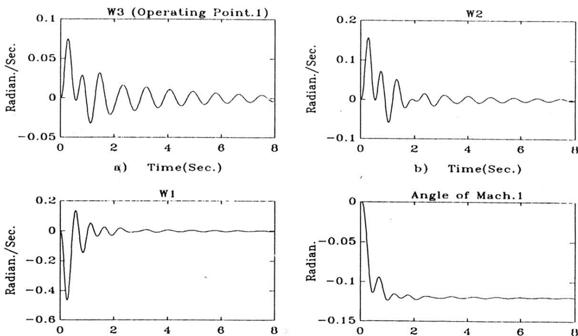
شکل (۴-۱۱) منحنی های تغییرات سرعت ماشینهای سنکرون و زاویه ماشین آ در نقطه کار
