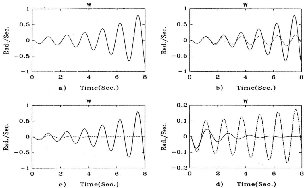
شکل (۵-۴) منحنی تغییرات سرعت بر حسب زمان در \chi=0.85
