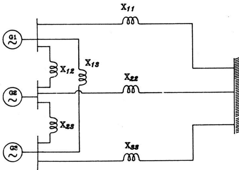
شکل (۹-۴) شبکه قدرت مورد مطالعه
