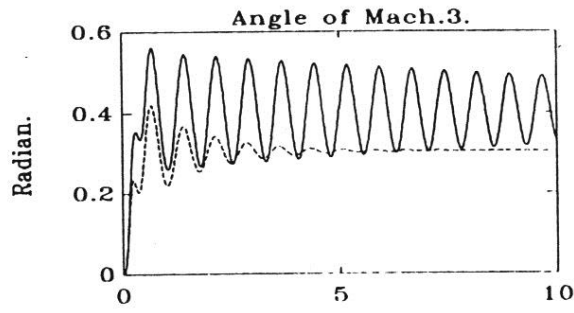
شکل (۲-۵) منحنی های تغییرات سرعت ماشینهای سنکرون و زاویه ماشین ۳ در حالتی که سیگنال کنترل ماشین ۳ قطع شده است (کنترل بهینه معمولی —، کنترل بهینه بر اساس مجموعه ای از نقاط کار ---)
