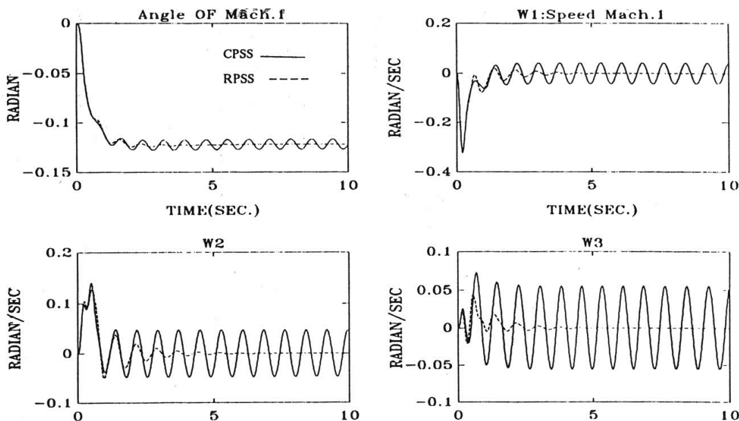
شکل (۴-۱۵) منحنی تغییرات سرعت ماشینهای سنکرون و زاویه ماشین ۱ در نقطه کار
