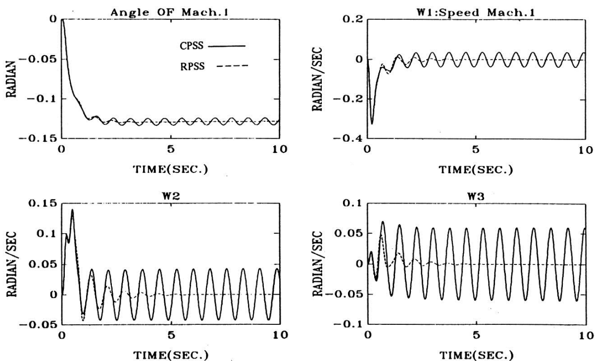
شکل (۴-۱۶) منحنی های تغییرات سرعت ماشینهای سنکرون و زاویه ماشین ۱ در نقطه کار ۶ جدول (۴-۱۳) با کنترل کننده های CPSS و RPSS
