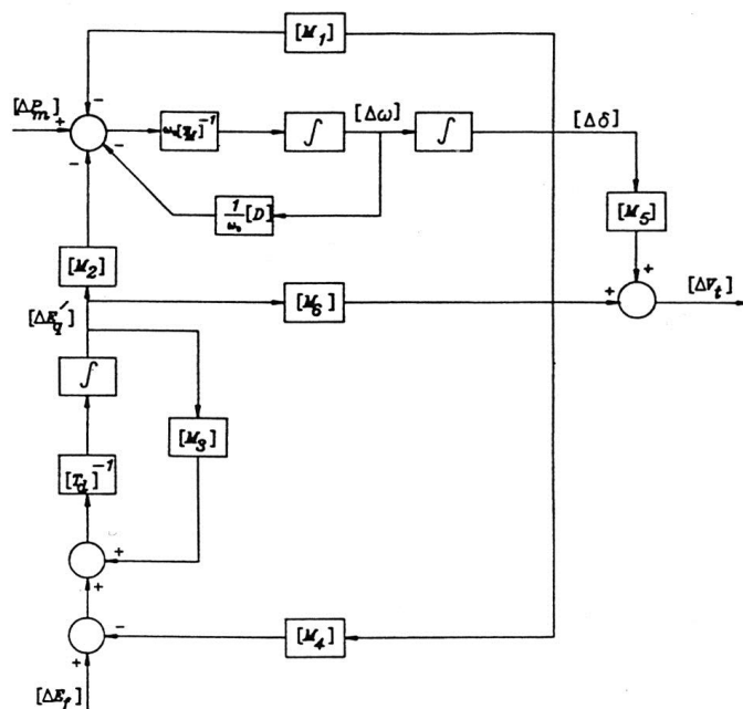
شکل (۷-۴) بلوگ دیاگرام مدل تعمیم یافته هفرون فیلیپ
