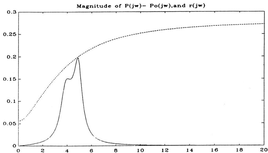
شکل (۲-۴) تابع حداکثر عدم قاطعیت متناظر با X=1.5
