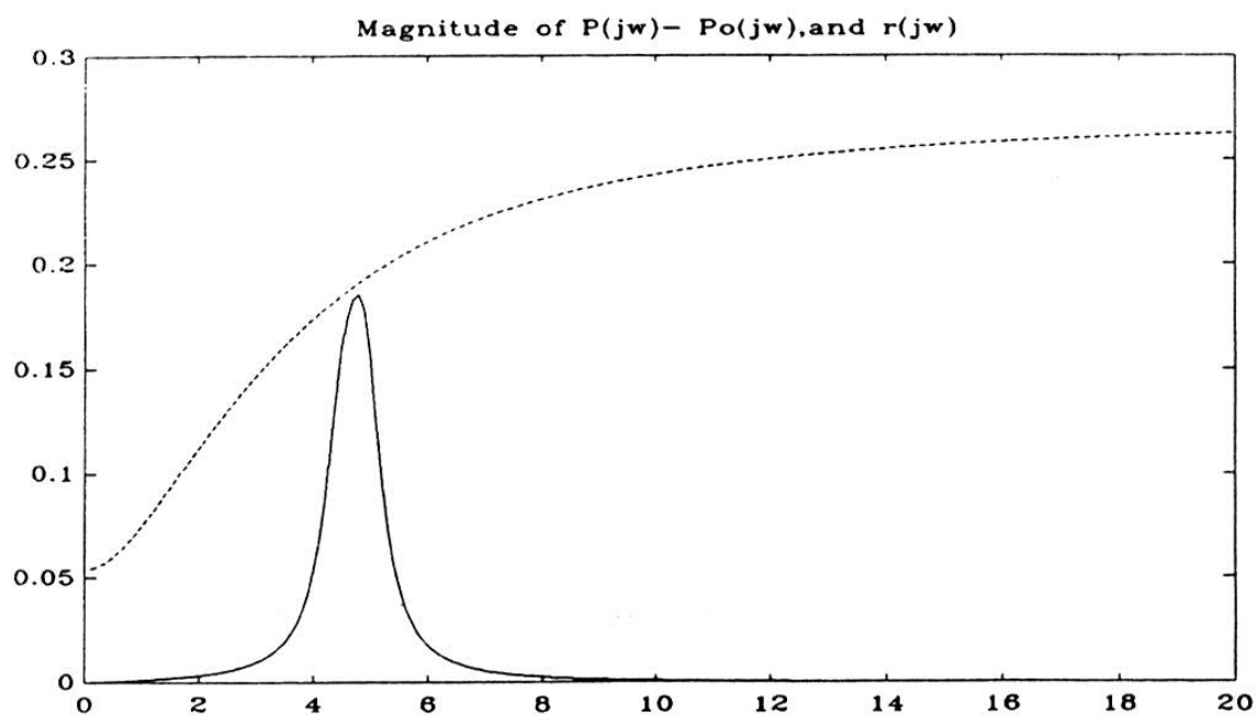
شکل (۳-۴) تابع حداکثر عدم قاطعیت متناظر با X=1.2
