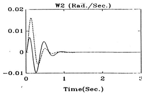
شکل (۲-۵) منحنی های تغییرات سرعت ماشینهای سنکرون و زاویه ماشین ۳ در حالتی که سیگنال کنترل ماشین ۳ قطع شده است (کنترل بهینه معمولی —، کنترل بهینه بر اساس مجموعه ای از نقاط کار ---)
