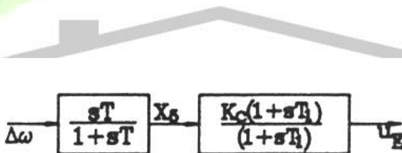
شکل (۳-۲) - بلوک دیاگرام PSS
