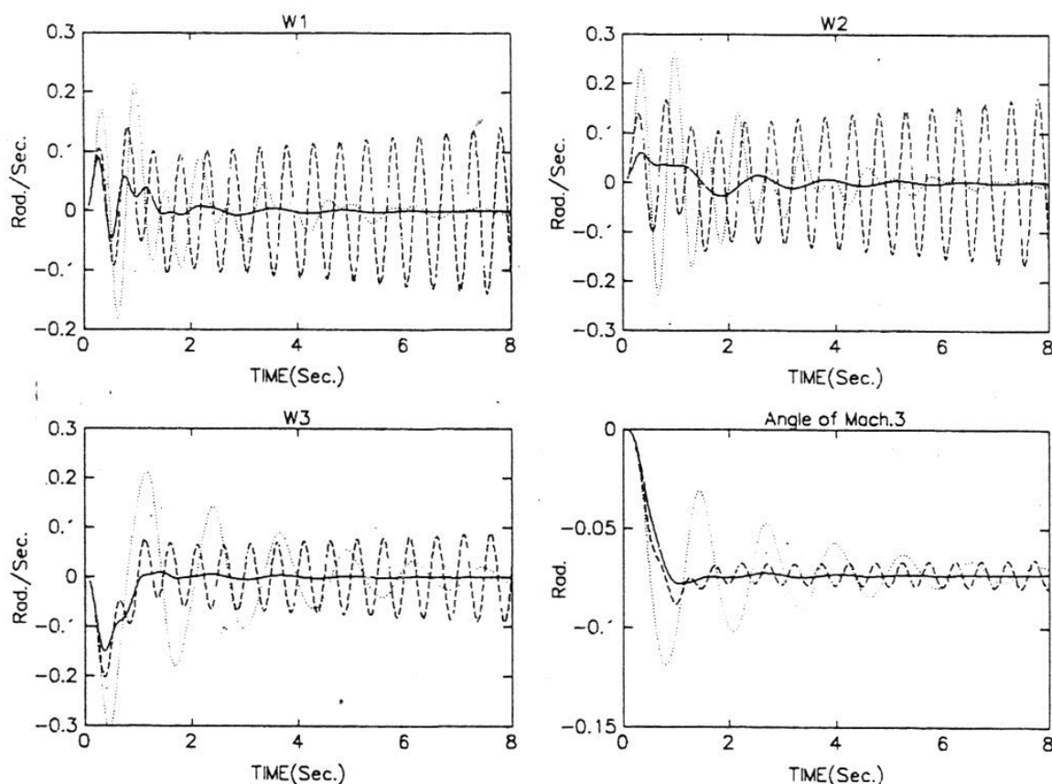
شکل (۱-۵) منحنی های تغییرات سرعت ماشینهای سنکرون و زوایه ماشین ۳
