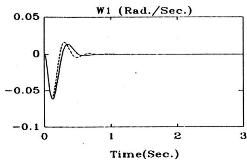
شکل (۲-۵) منحنی های تغییرات سرعت ماشینهای سنکرون و زاویه ماشین ۳ در حالتی که سیگنال کنترل ماشین ۳ قطع شده است (کنترل بهینه معمولی —، کنترل بهینه بر اساس مجموعه ای از نقاط کار ---)
