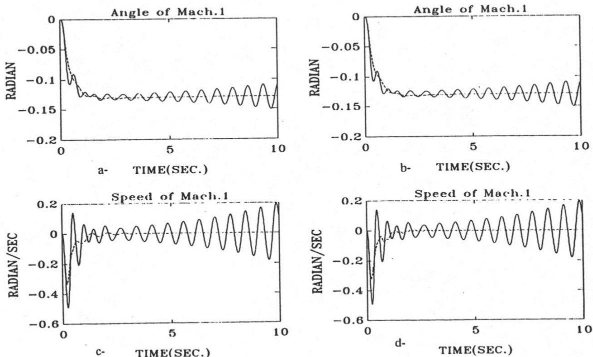
شکل (۴-۱۴) منحنی تغییرات و زاویه ماشین ۱.
