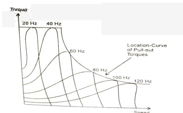
شکل (۱۱-۳) مشخصه گشتاور سرعت موتورهای القائی با کنترل ولتاژ و فرکانس
