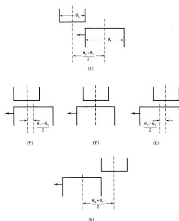
موقعیت‌های رتور ۱- اندوکتانس به‌طور خطی از این موقعیت افزایش می‌یابد. ۲-۳- موقعیت‌های اندوکتانس حداکثر ۴- وقتی رتور از این موقعیت حرکت می‌کند اندوکتانس به‌طور خطی کاهش می‌یابد. ۵-۴ در مقابل \theta
