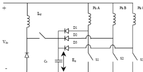
Fig. 7. C-dump Converter
