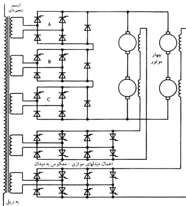
طرح اصلی یک آرایش تریستوری برای لوکوموتیو
