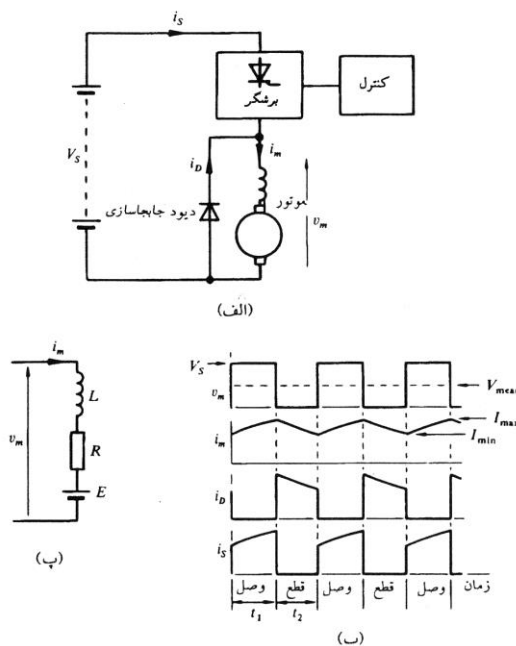
موتور تغذیه شده با برشگر. مدار، (الف) مدار، (ب) شکل موجها، (پ) مدار معادل تقریبی
