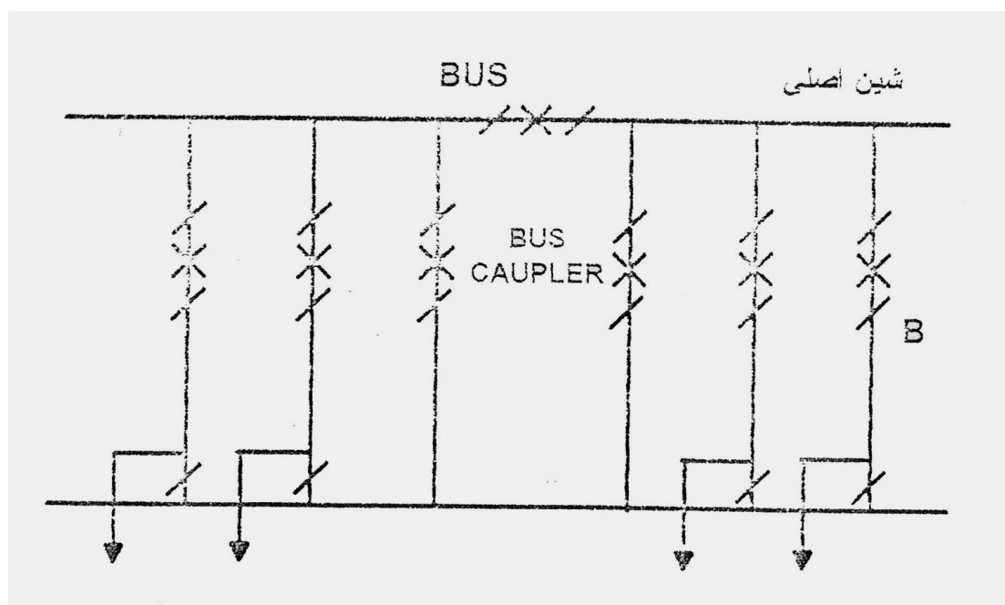
بوس بار دوبل (اصلی و رزرو)
