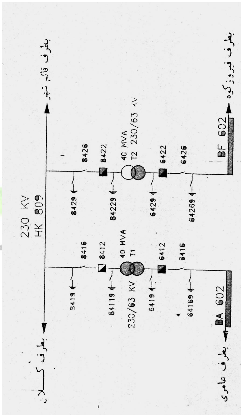
۱-۲-۲ شین بندی ساده تک شینه
