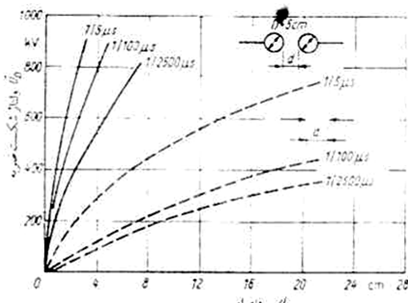
شکل (۲۴-۳) ولتاژ شکست روغن را برحسب فاصله برای ولتاژ ضربه با نیم زمانهای پشت مختلف نشان می دهد
