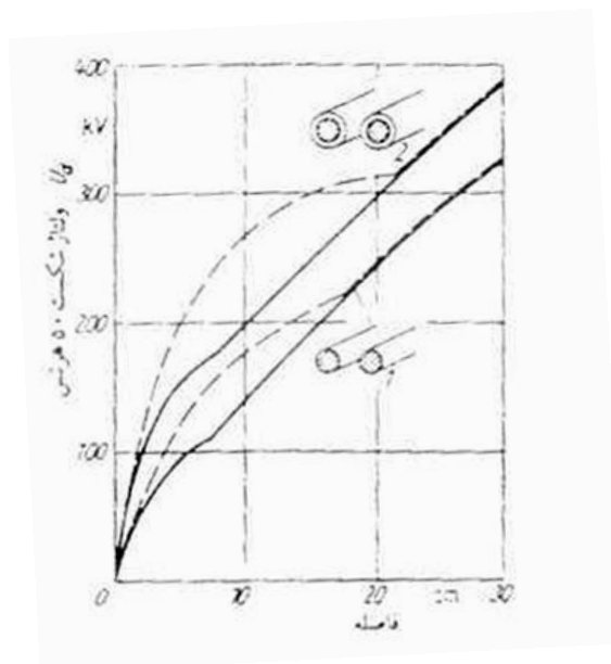
شکل (۲۹-۳) ولتاژ شکست برای الکترودهای استوانه - استوانه بدون عایق (لخت) و عایق شده با دو ورقه عایق نشان می
