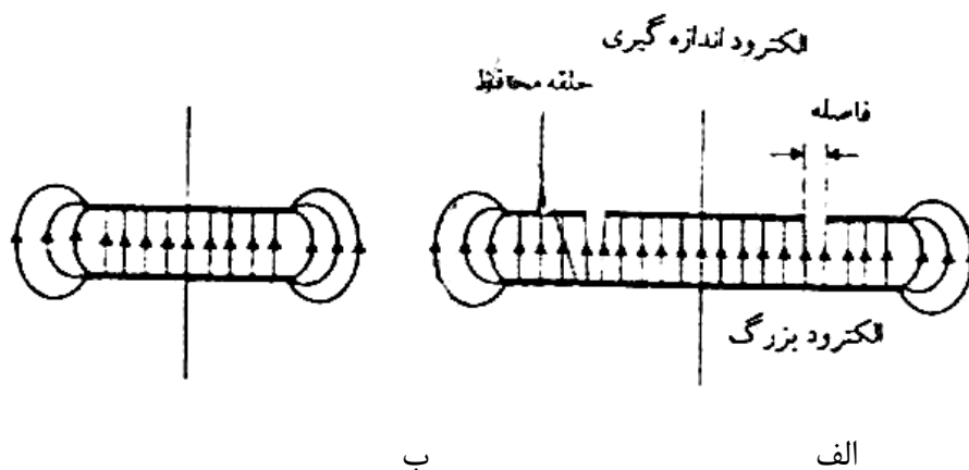
شکل (۱۰-۲): الف) خازن صفحه ای با حلقه محافظ ب) بدون حلقه محافظ
