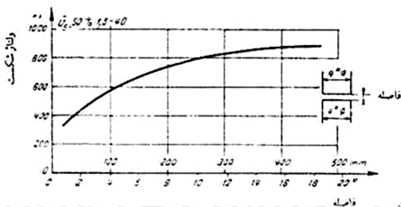
شکل (۳-۴۲): ولتاژ شکست بر حسب فاصله در روغن ترانسفورماتور برای ولتاژ ضربه 1/5/40 میکروثانیه بین الکترودهای
