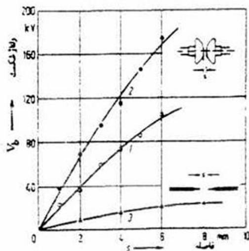
شکل (۱۷-۳): ولتاژ شکست برای الکترودهای مختلف
