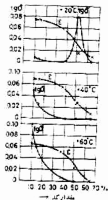
شکل ۱۲-۱- tgδ و ε در تابعیت از مقدار کلر
