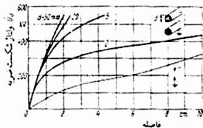
شکل (۳-۲۳) ولتاژ شکست الکترودهای کره - صفحه و استوانه - استوانه موازی
