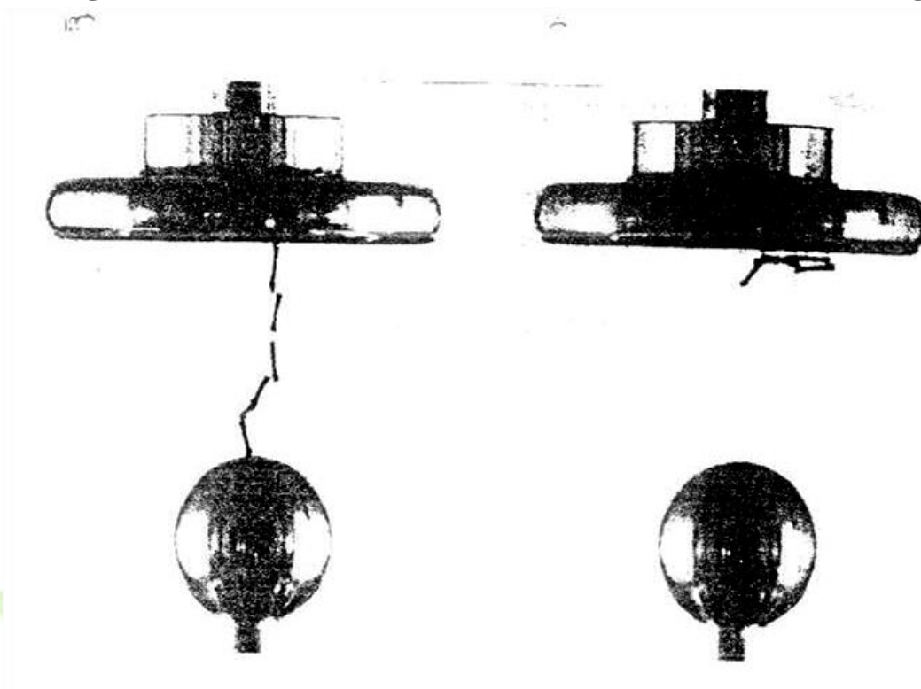
شکل (۳-۳): اثر ذرات معلق در روغن عایق و بوجود آمدن پل
