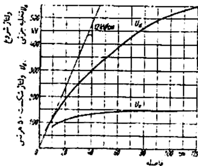
شکل (۳-۴) تغییرات ولتاژ شکست برای روغن ترانسفورماتور بر حسب فاصله در فرکانس ۵۰ هرتس
