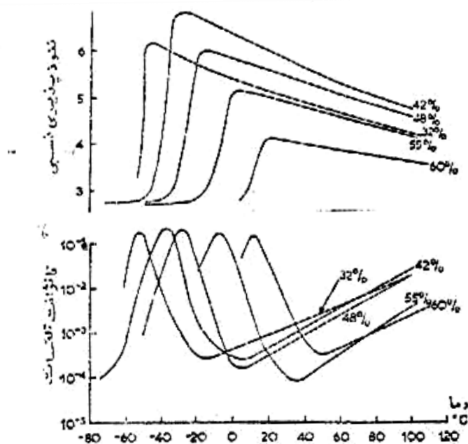
شکل (۱۳-۱) تغییرات نفوذ پذیری نسبی و ضریب تلفات دی فنیل های کلرینه شده نسبت به دما
