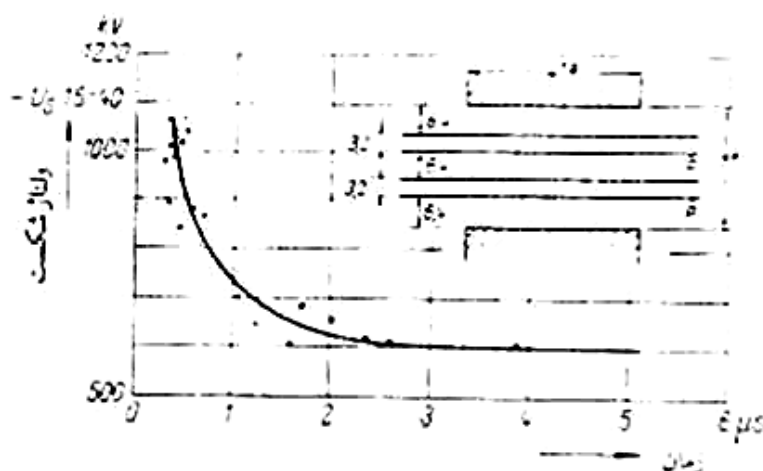
شکل (۳-۴۳): زمان تأخیر شکست بین الکترودهای استوانه ای با قطر ۴ اینچ (حدود ۱۰ سانتی متر) در روغن
