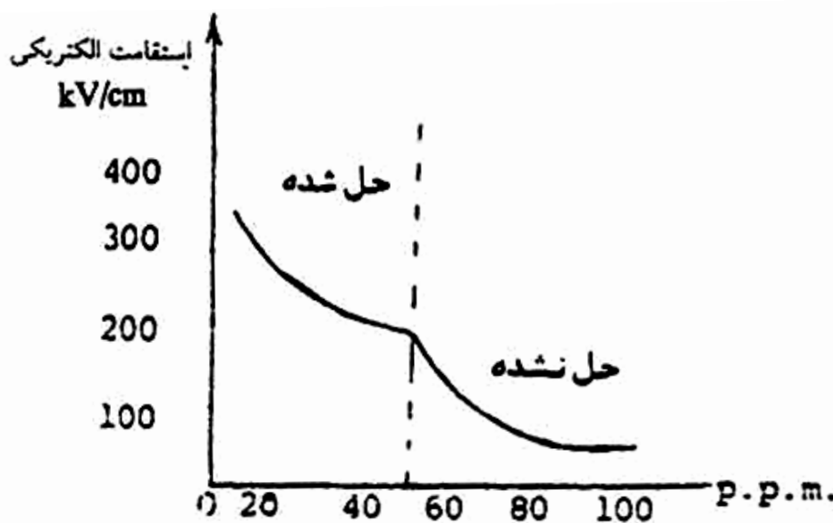
شکل (۸-۳) تغییرات ولتاژ شکست روغن با درصد آب حل شده در آن
