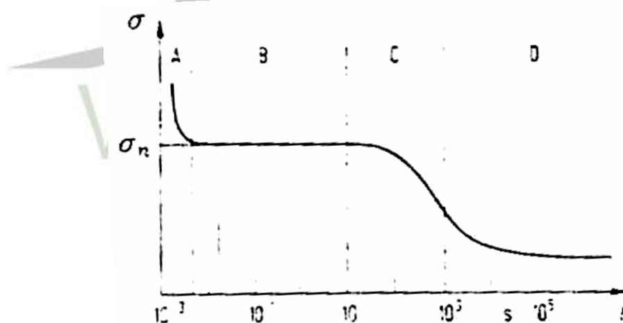
شکل (۲-۹) : تغییرات ضریب قابلیت هدایت الکتریکی یک عایق مایع برحسب زمان
