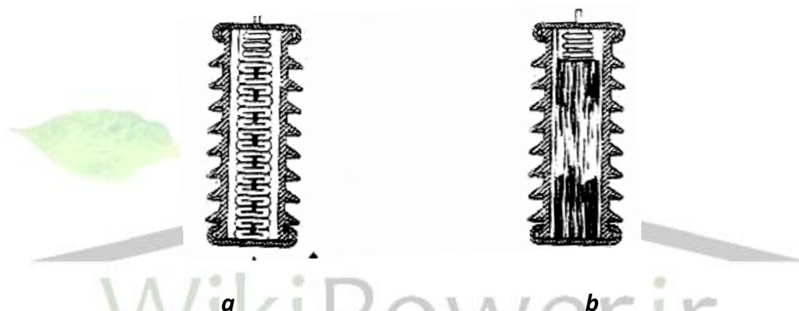
شکل ۹-۱- خازن استوانه شکل، کاغذ - روغن شکل ۱۰-۱- خازن مسطح کاغذ - روغن
