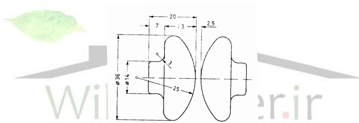
شکل (۱۶-۲): ابعاد الکترودهای عرق چین کروی برای تعیین ولتاژ شکست عایق مایع
