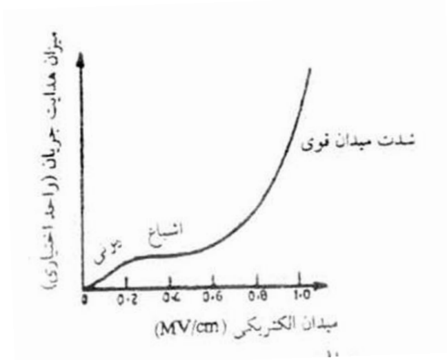
شکل (۳-۱) مراحل مختلف هدایت عایق های مایع
