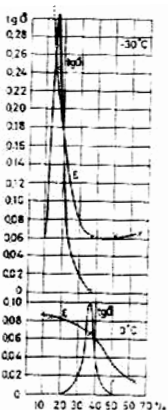
شکل ۱۱-۱- ضریب تلفات tgδ و ε در تابعیت از مقدار کلر
