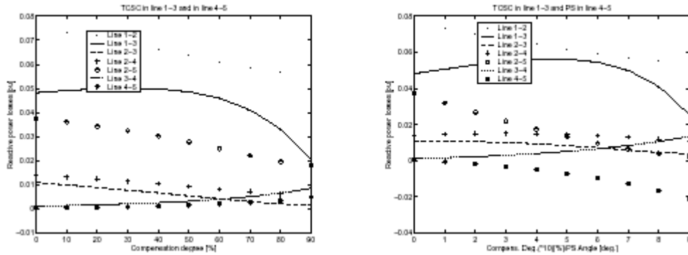
تصویر ۴۷- افت واکنشگر برای شبکه Hale
