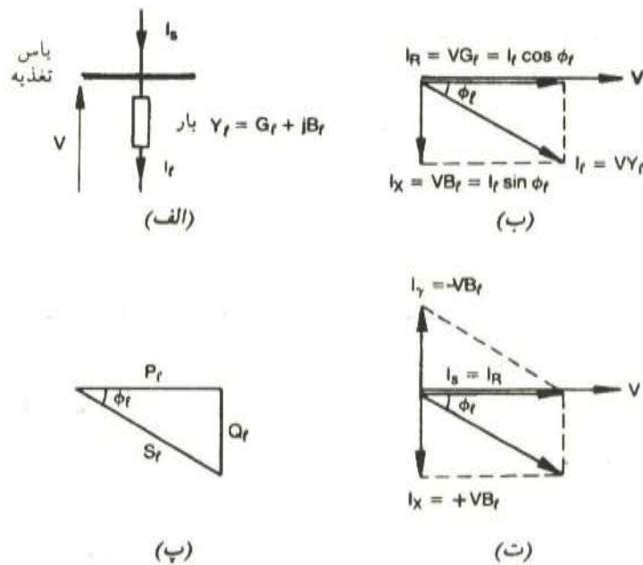
شکل ۱- الف الی (ت) اصلاح ضریب توان
