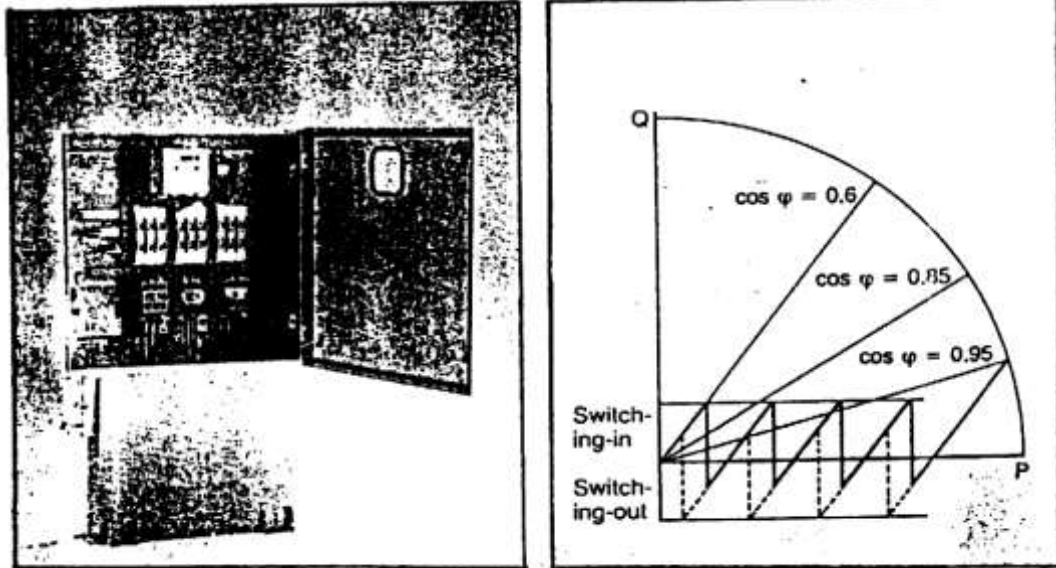
شکل ۱۹- بانک خازن اتوماتیک
