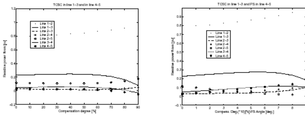
تصویر ۴۵- جریانهای برق واکنشگر برای شبکه Hale
