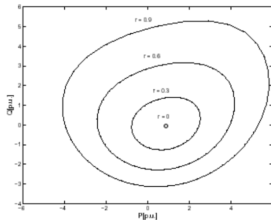
تصویر ۳۵- تغییرات Q در برابر P در خط ۵-۵
