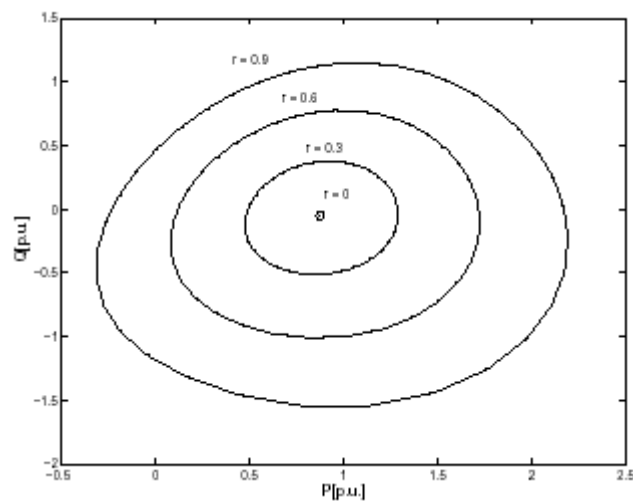
تصویر ۳۵- تغییرات Q در برابر P در خط ۵-۵
