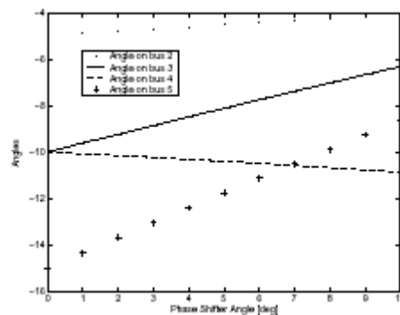
تصویر ۲۱- زاویای ورودی ناقلان در PS واقع در خط ۴-۵
