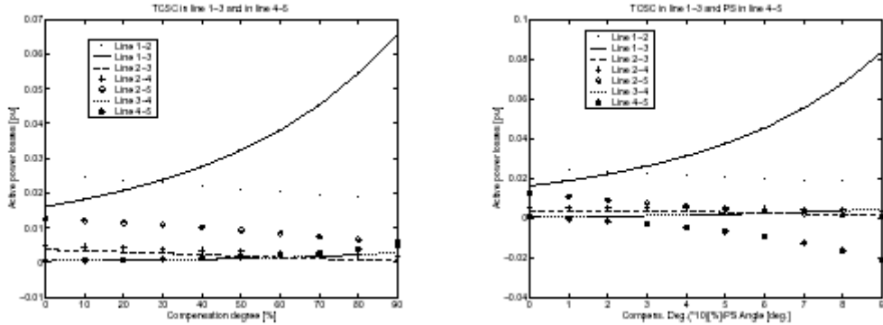
تصویر ۴۶- افت کنشگر برای شبکه Hale
