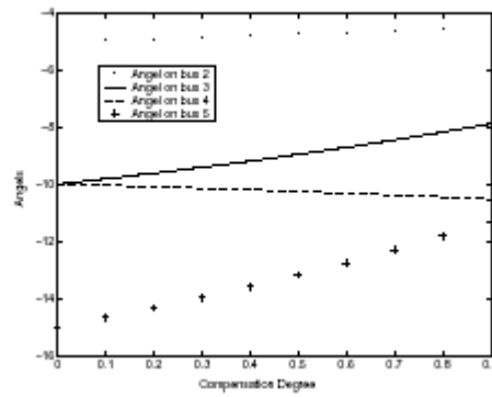
تصویر ۹- زاویای روی ناقلان برای TCSC واقع در خط ۴-۵ ( حالت دوم - مدل تزریقی )
