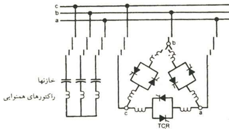
شکل ۸ ب- TCR سه فاز همراه با خازن های موازی
