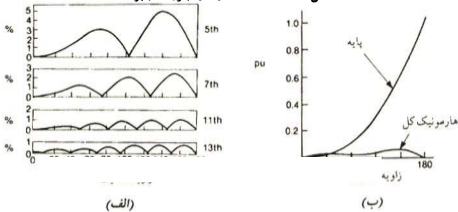
شکل ۷- مشخصات ولتاژ جریان جبران کننده TCR
