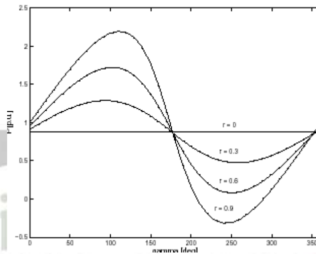
تصویر ۳۲- تغییرات p در برابر \gamma در خط ۴-۵
