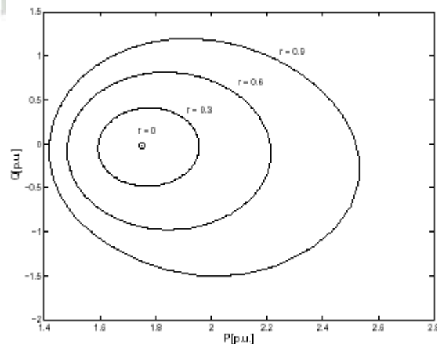
تصویر ۳۸- تغییرات Q در برابر P در خط ۴-۱
