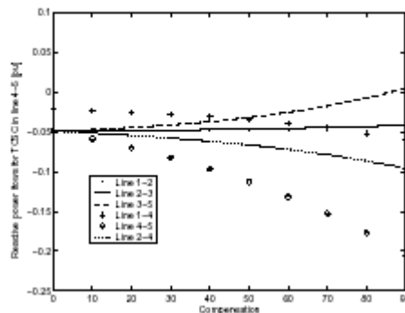
تصویر ۱۲- جریان برق واکنشگر برای TCSC واقع در خط ۴-۵ ( حالت اول )
