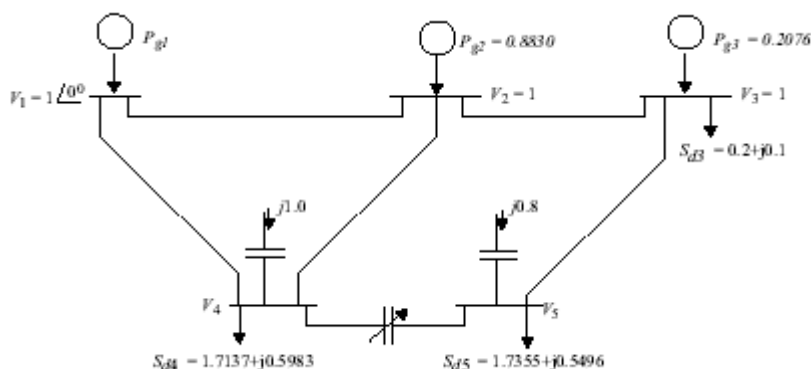
تصویر ۵ - سیستم ۵ ناقلی
