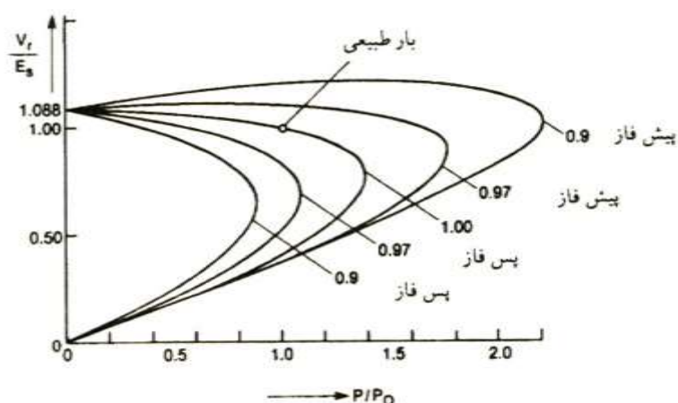
شکل ۴- مقدار ولتاژ انتهای خط در یک خط شعاعی ۲۰۰ مایل بدون تلفات
