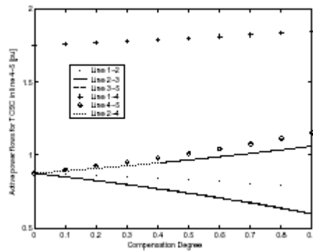
تصویر ۱۱- جریان برق فعال برای TCSC واقع در خط ۴-۵ ( حالت دوم - مدل تزریقی )
