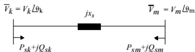
تصویر ۳۰- مدل تزریقی برای UPFC
