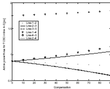
تصویر ۱۰- جریان برق فعال برای TCSC واقع در خط ۴-۵ ( حالت اول - واکنشگر متغیر )
