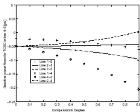
تصویر ۱۳- جریان برق واکنشگر برای TCSC واقع در خط ۴-۵ (حالت دوم)
