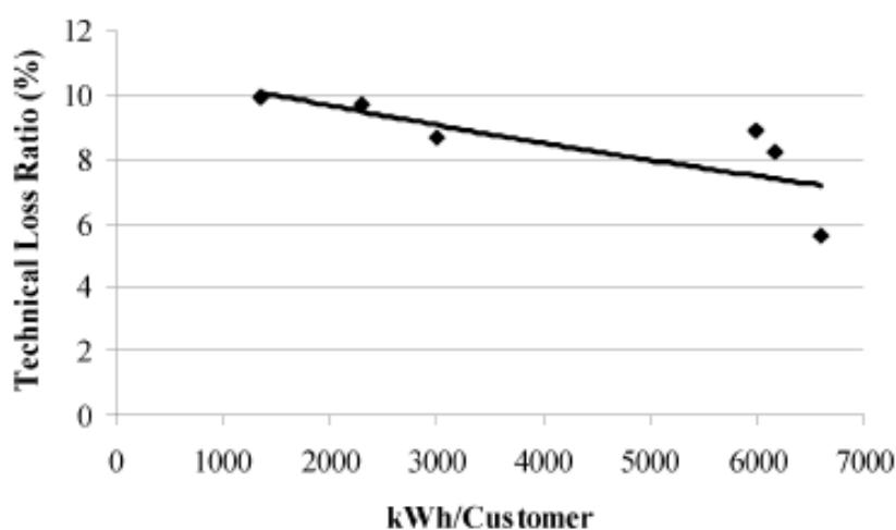
شکل ۷-۷: نرخ تلفات تکنیکی بر حسب کیلووات ساعت بر مشترک
