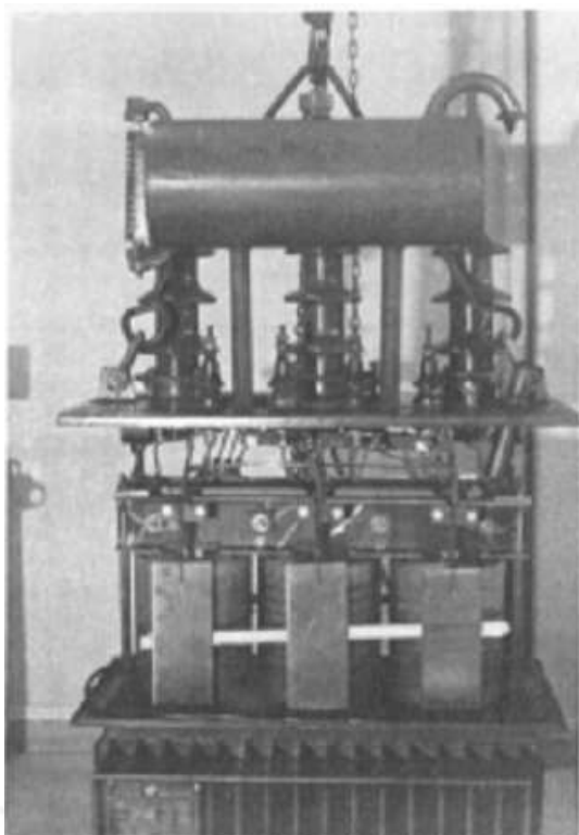
شکل ۲-۳: نمایش نصب شیلدهای مسی در پیشانی سی پیچی ها و در حد فاصل سی پیچی ها و بدنه مخزن
