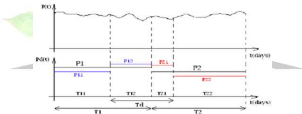
شکل ۷-۲: پروفیل بار و مقدار مصرف انرژی یک مشترک طی ۲ ماه
