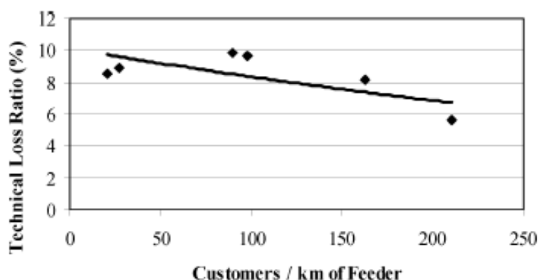
شکل ۶-۷: نرخ تلفات تکنیکی بر حسب تعداد مشترکین بر کیلومتر فیدر
